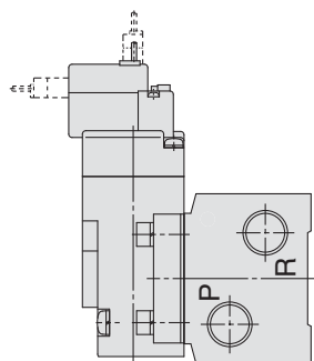
VVEX2-1 (Internal pilot)
