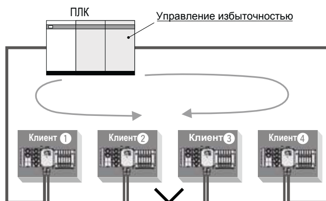
Поток данных при разъединении кабеля
