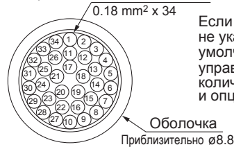
34 провода Кабель
